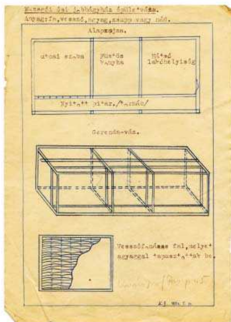
9. Mozsgói jobbágyház épületváza. Kovács József Pozsonyi u. 5. sz. háza
